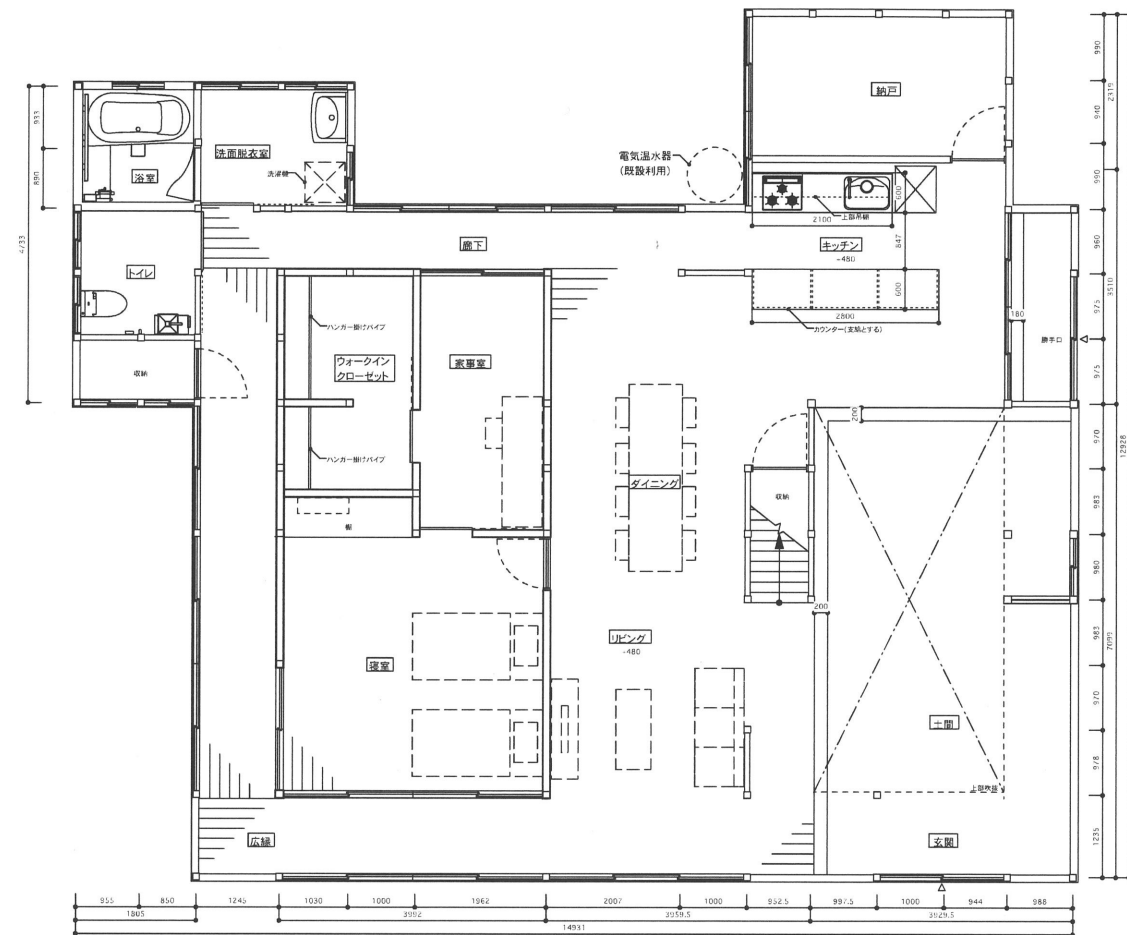
1階平面図
